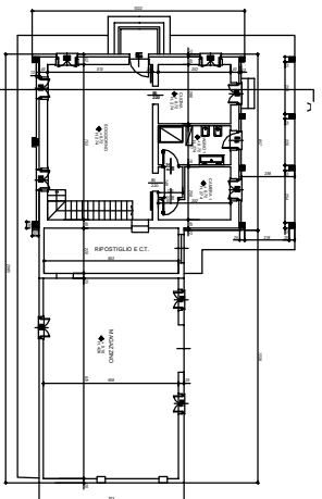
PIANTA PIANO TERRENO
